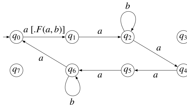
Figura 6.6: Autômato subjacente após a execução do algoritmo 6.1
