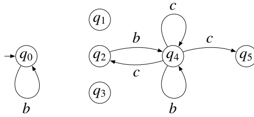
Figura 6.2: Autômato após a execução das ações elementares
