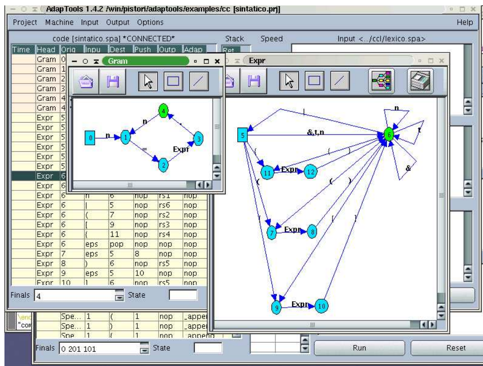
Figura 11.1: Meta-reconhecedor Wirth para AdapTools
