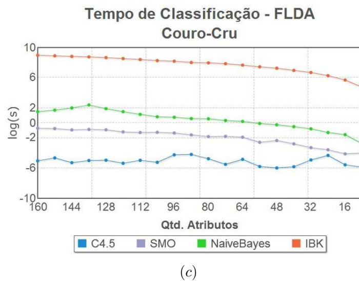
Figura 6.5: Comportamento do classificador, (a) classificação correta(%), (b) tempo de treinamento em \log_2(s) , (c) tempo de classificação em \log_2(s) .
